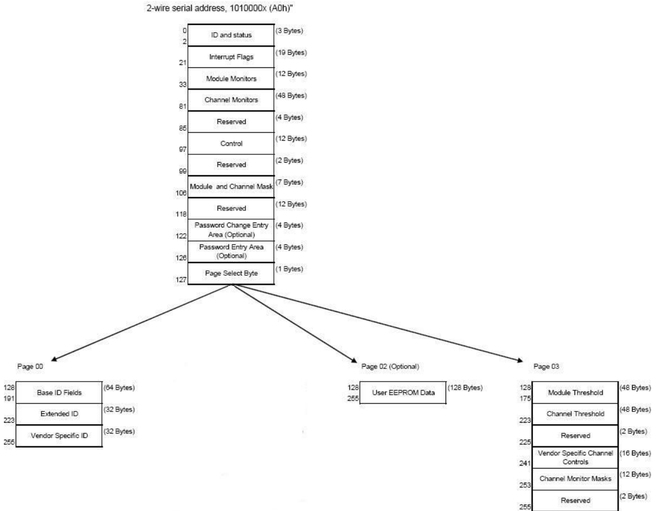
Figure4. QSPF Memory Map
